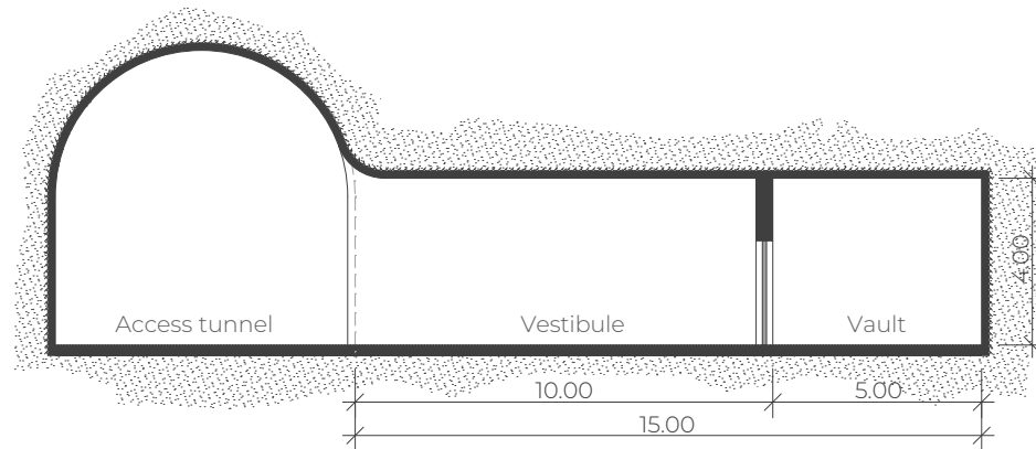
Longitudinal section
